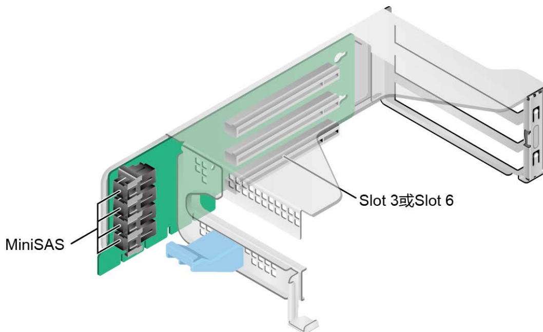
图3-21 Riser 卡 5 (SAS Riser)
