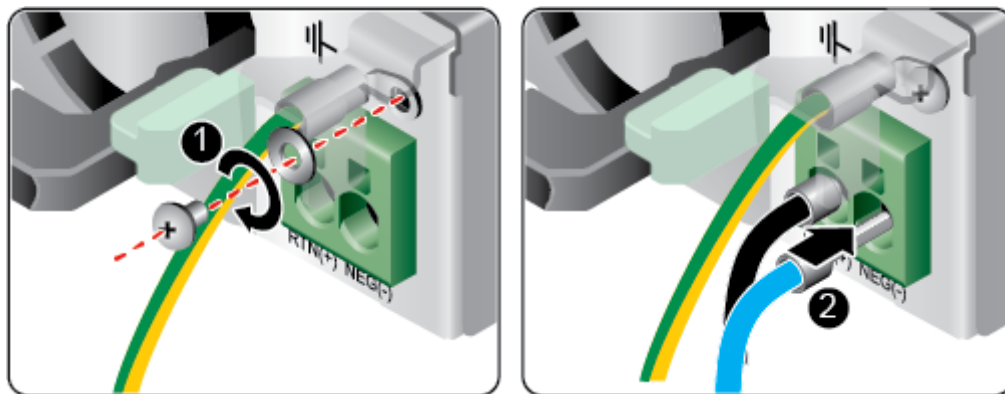
图6-19 连接线缆
