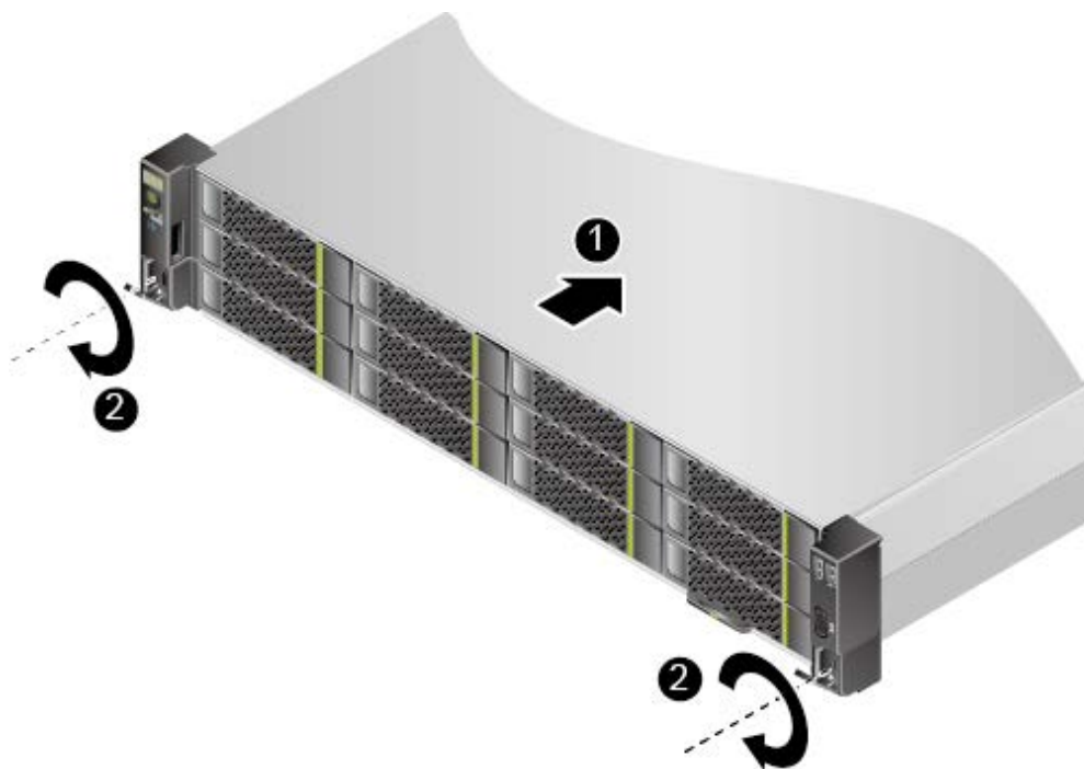
图6-9 安装服务器
