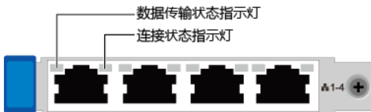
图3-9 TM210（4*GE 电口）
