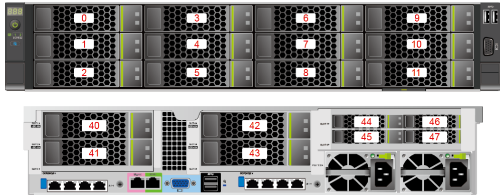
图3-11 12x3.5 英寸硬盘 EXP 配置硬盘编号
