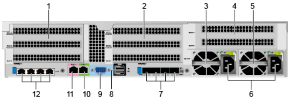
图3-7 后面板组件
