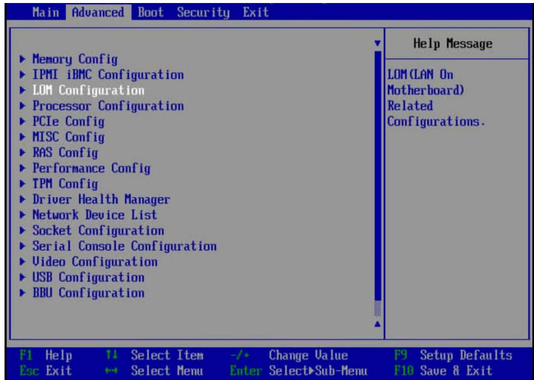
图6-35 “Advanced”界面
