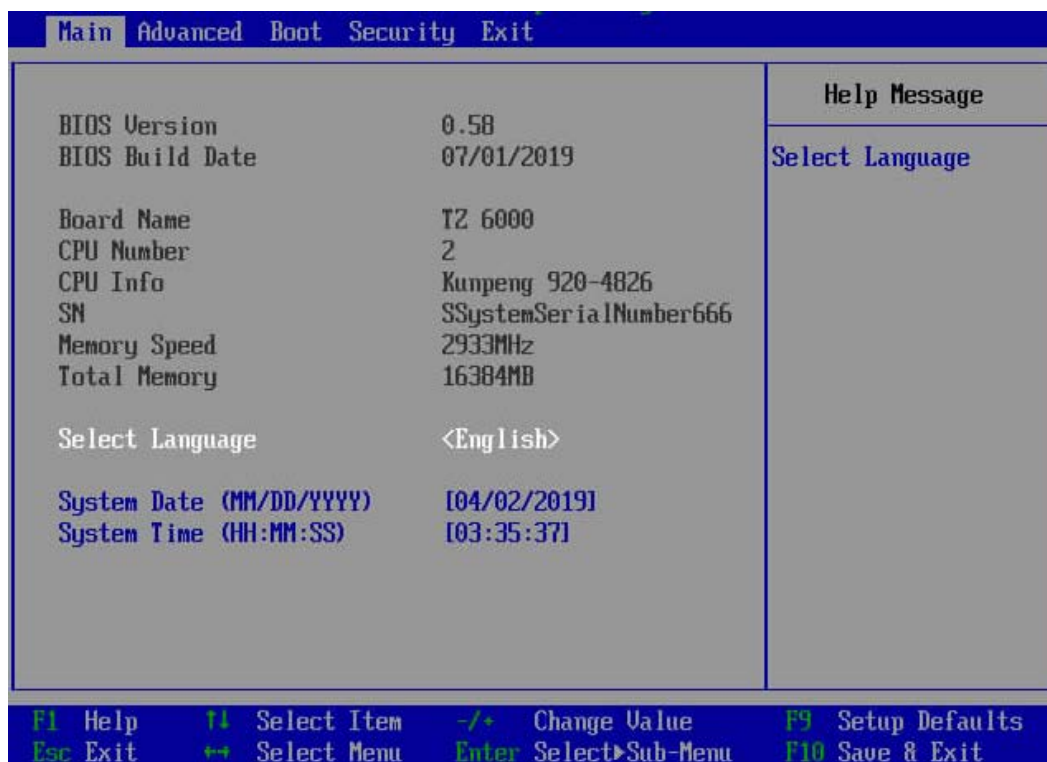
图6-38 “Main”界面
