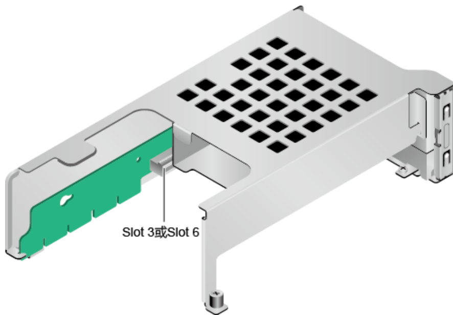
图3-20 Riser 卡 4（1x16）
