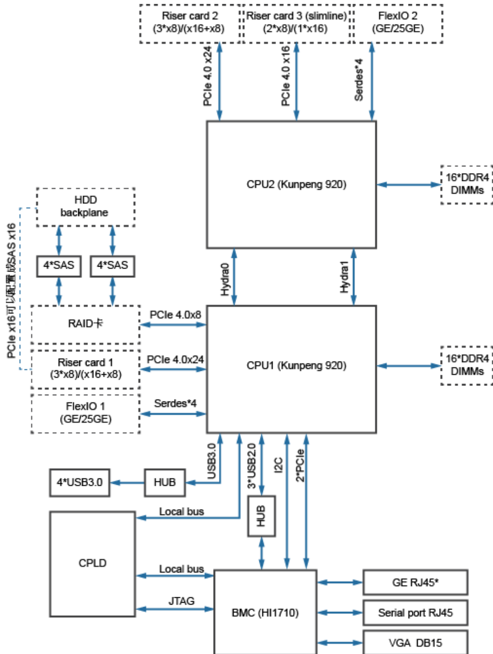
图2-3 R3820 G3 逻辑结构
