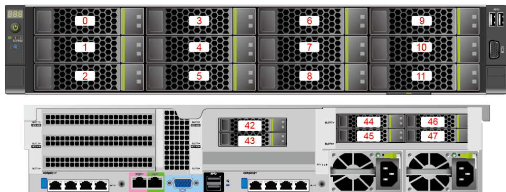
图3-12 12x3.5 英寸硬盘直通配置
