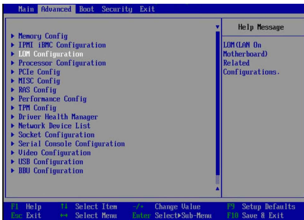
图6-34 “Advanced”界面
