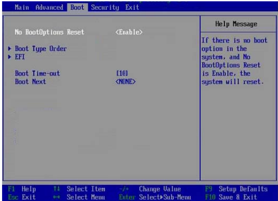
图6-33 Boot 界面
