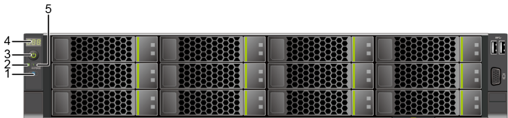
图3-4 12x3.5 英寸硬盘配置前面板指示灯和按钮
