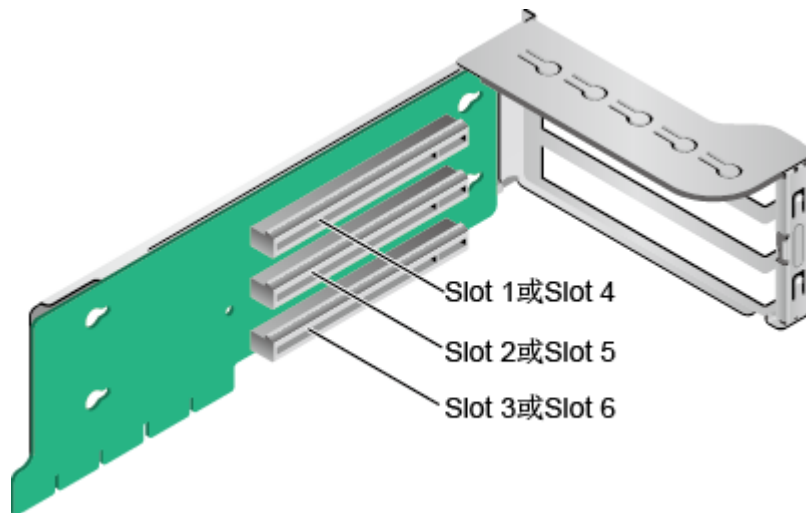
图3-17 Riser 卡 1 (3x8)
