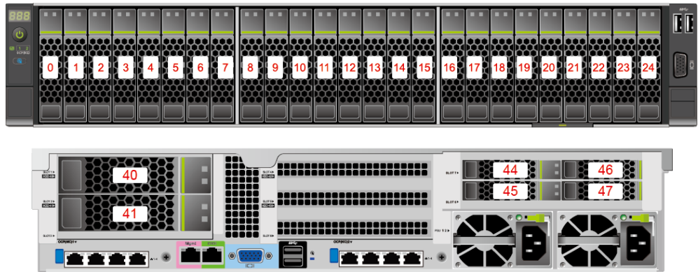
图3-13 25x2.5 英寸硬盘 EXP 配置硬盘编号
